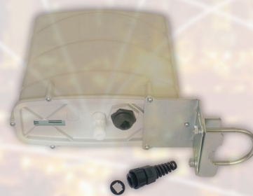
IDA000103 Sensore di particolato PM10, PM4, PM2.5, PM1 (Ethernet)
